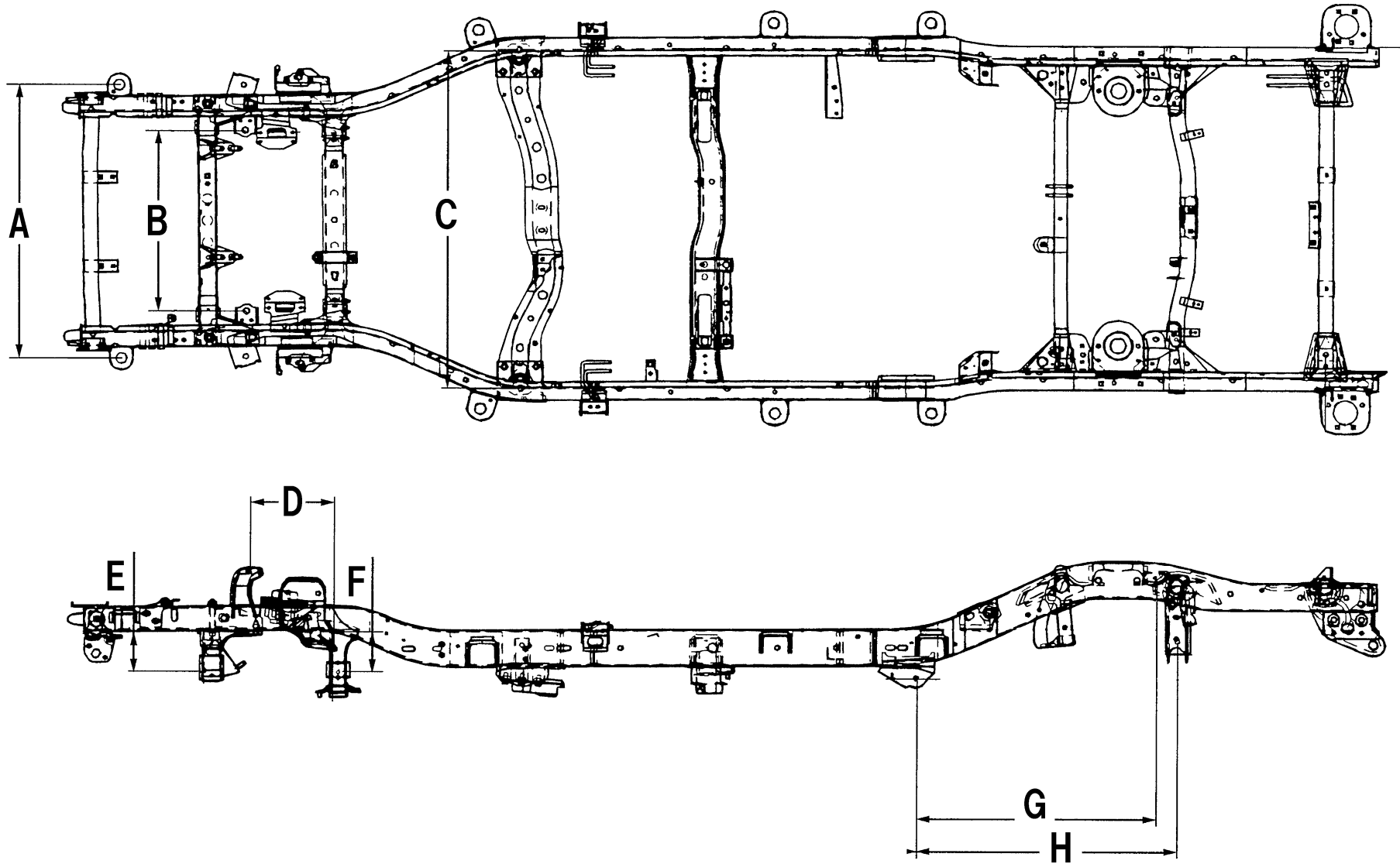
平面投影寸法図
