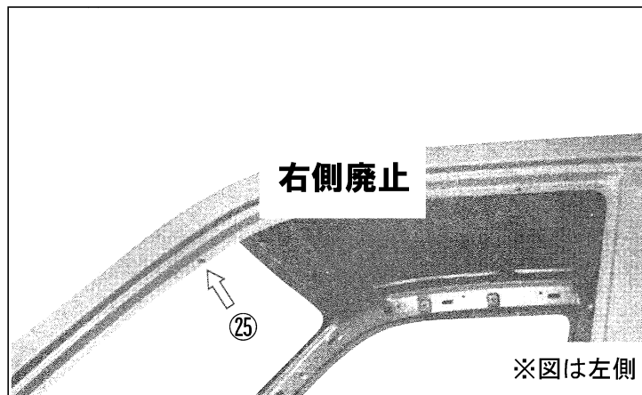
②⑤: リーンホースフロントピラーアッパーゲージホール
