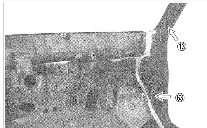
⑬: フロントピラーインナーアッパーゲージホール 8φ ⑥③: フロントピラーインナーロアゲージホール 8φ
