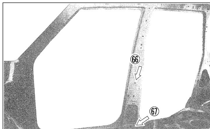
⑥⑥: クリップ穴 8φ ⑥⑦: リトラクター取付け穴 13φ
