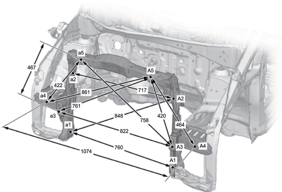
A5、a5 フロントバルクヘッドアッパフレーム 基準穴φ11
