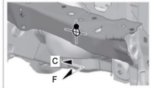
A5、a5 フロントバルクヘッドアッパフレーム 基準穴φ11
