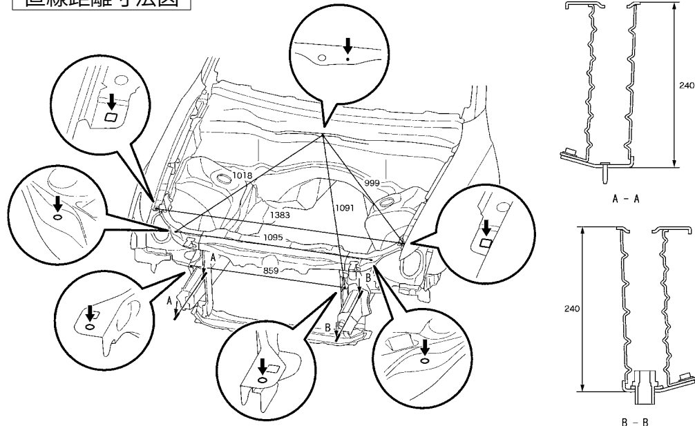
ポップアップフードリфта ASSY およびフードヒンジ取り付け部
