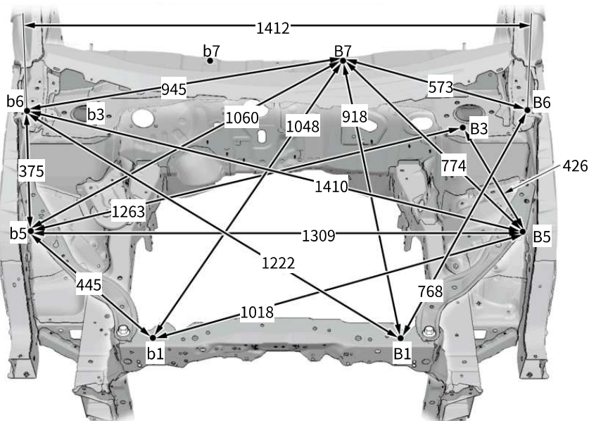
B7, b7 フロント ウィンドシールド ロア 基準穴φ12
