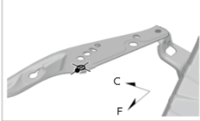
B5, b5 フロント フェンダ前部取付け穴φ7
