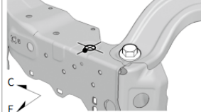
B1, b1 フロントバルクヘッド アップセンタ フレームA基準穴φ15
