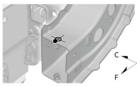
B2, b2 フロントバンパビーム取付け穴φ9
