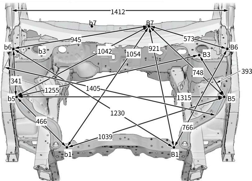
B7, b7 フロントウインドシールドロア 基準穴φ12
