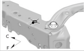
B1, b1 フード ストップ取付け穴φ10
